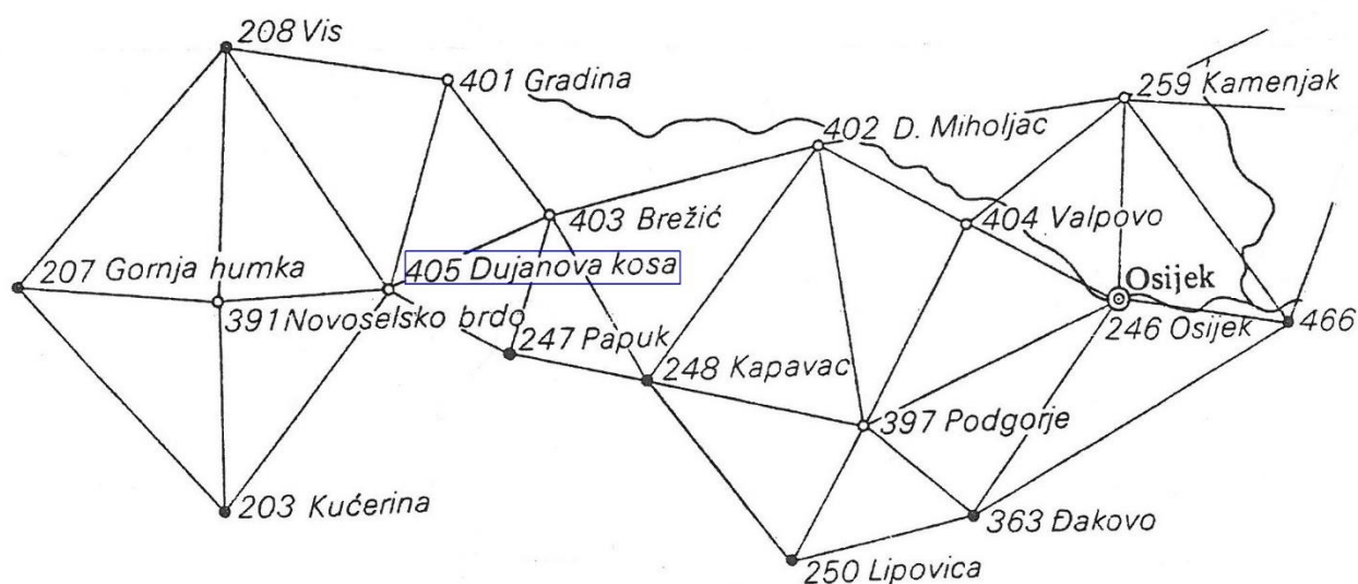
Slika 2. A-U trigonometrijska točka I. reda Petri vrh (gore) i novopostavljena 405 Dujanova kosa (dolje).
